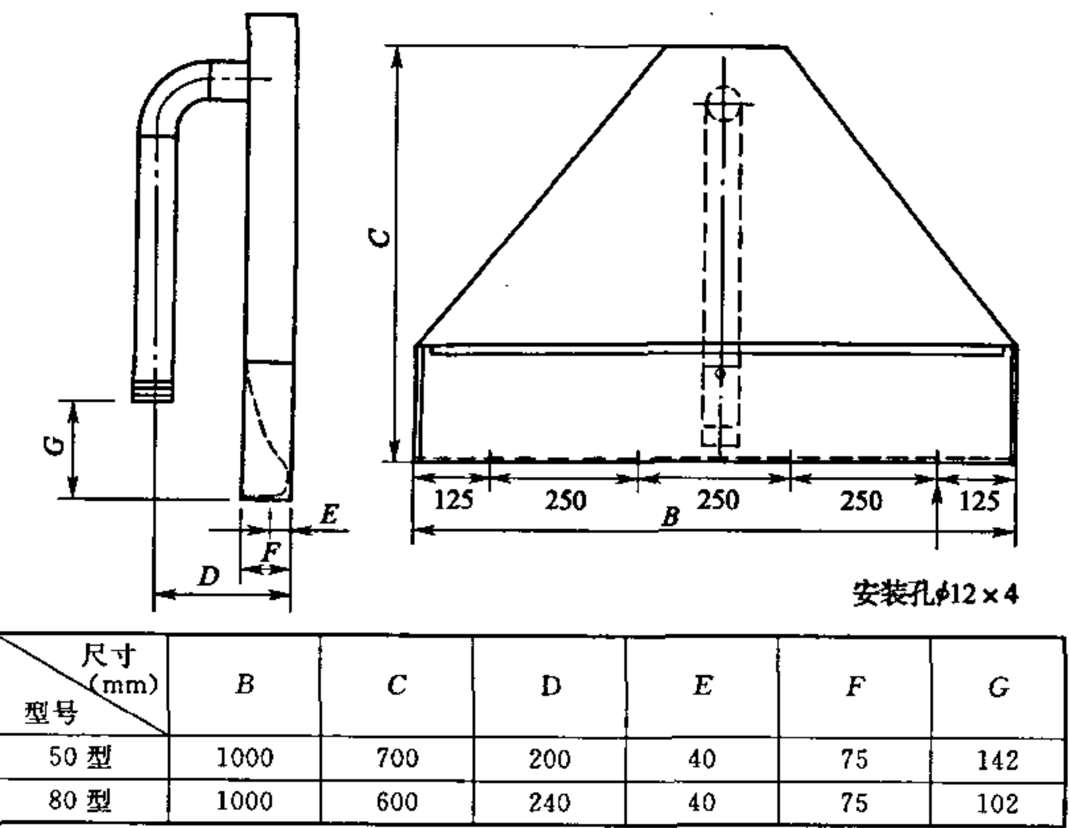
图 1 泡沫倾注器
